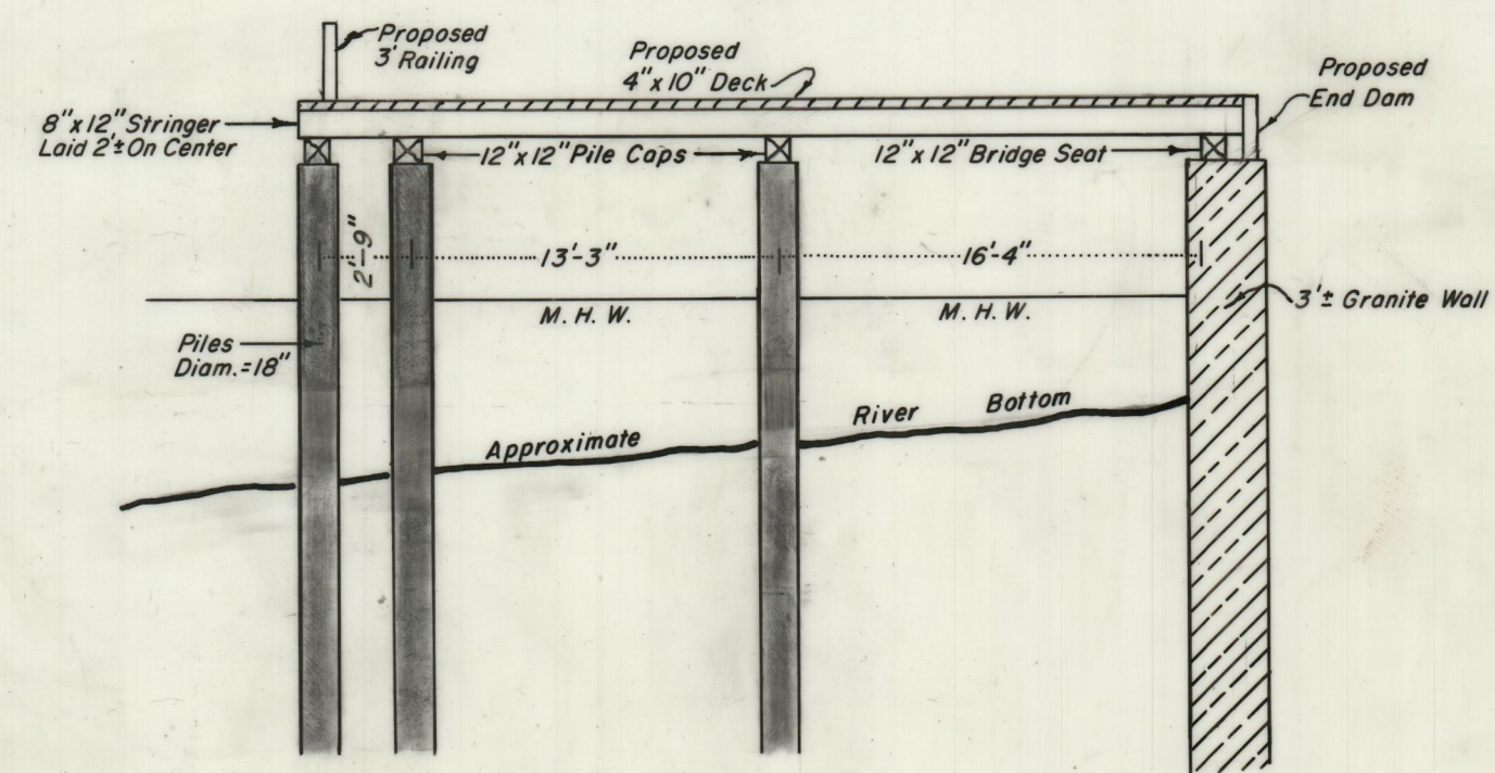
Section — A-A
